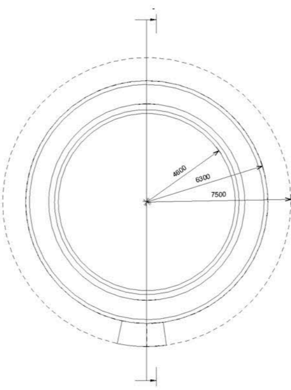
Plan 1:100
